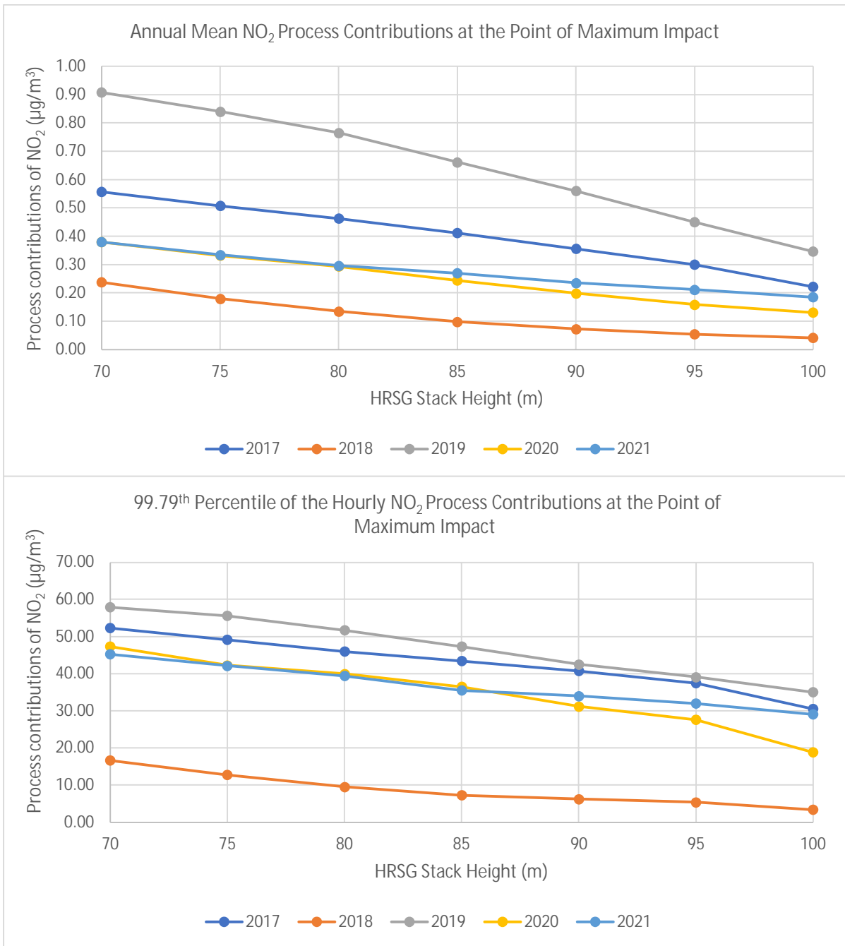
Figure 17 – Stack Height Assessment Graphs for the HRSG Stack
